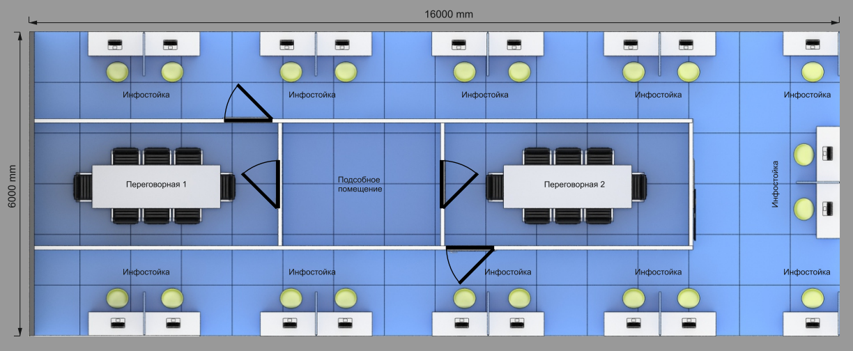
План стенда
